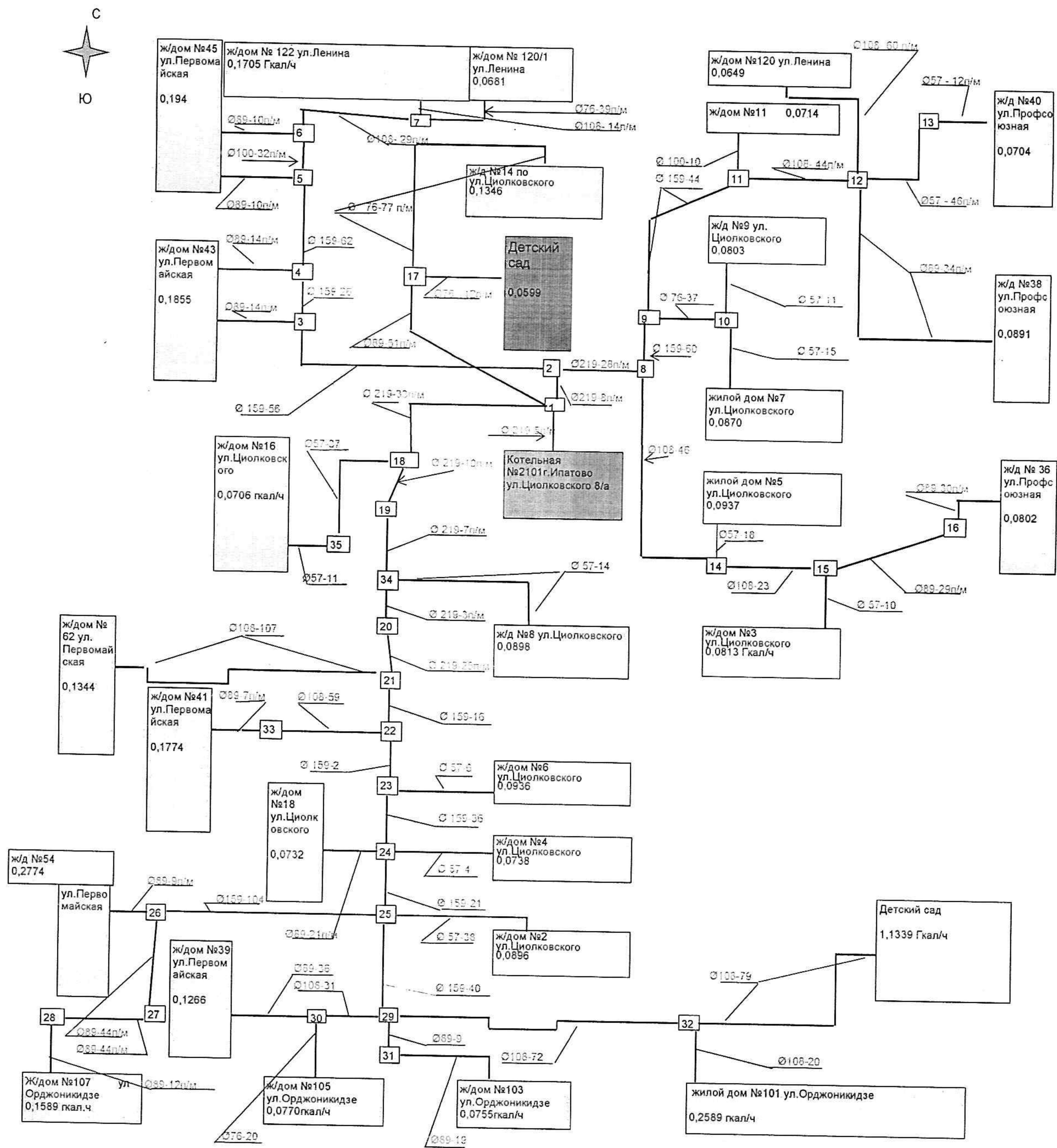
Схема теплосети котельная 2101 г.Ипатово
