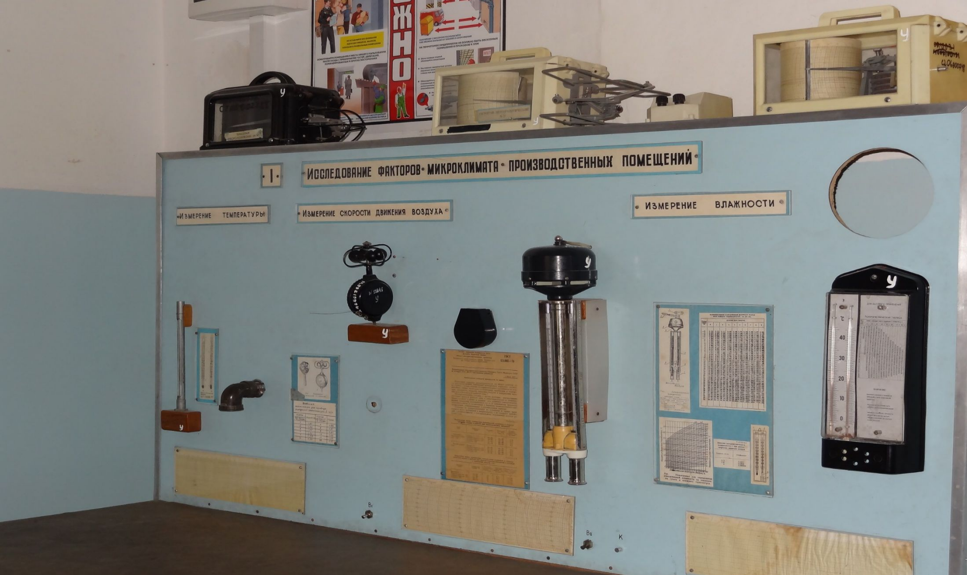
Стенд для исследований факторов микроклимата производственных помещений и выполнения практических работ по курсу «Охрана труда»
